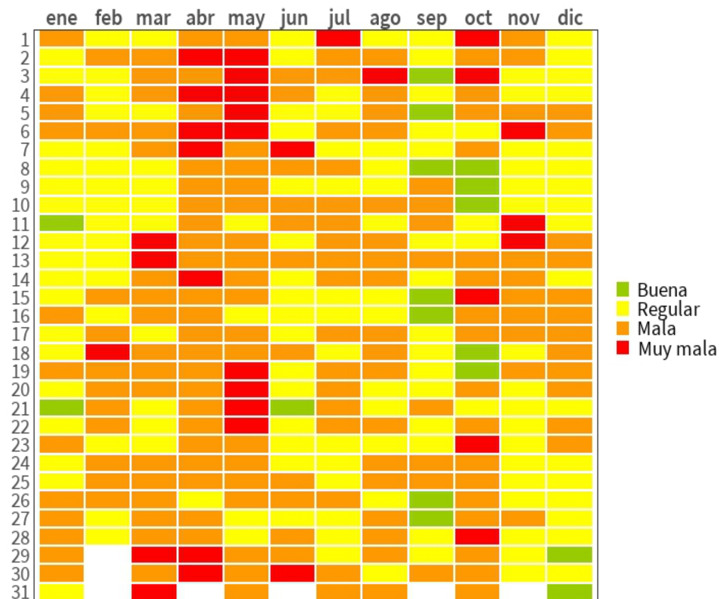
Calidad del aire por ozono
